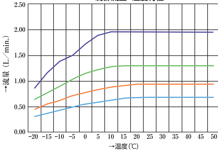
制御流量 温度特性
