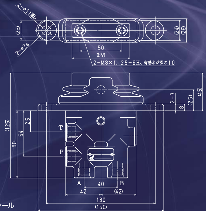
コントロールバルブ
