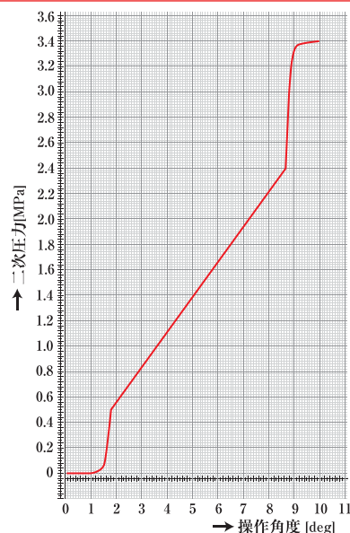
ストロークエンドで一次圧にショートするタイプ
