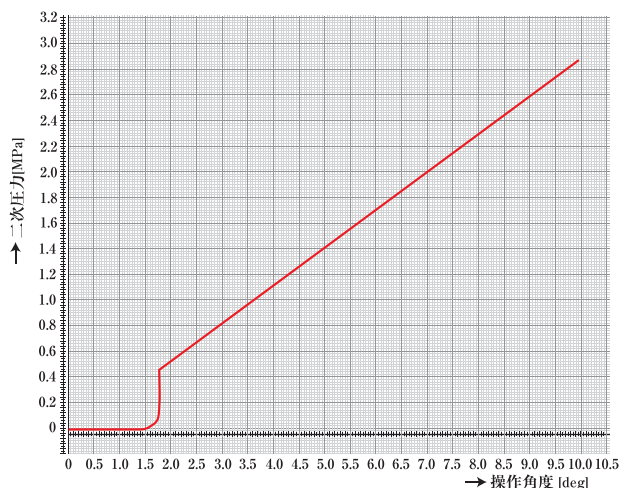
ストロークエンドまで二次圧を制御するタイプ
